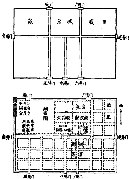
图：曹魏、后赵邺都北城复原略图
