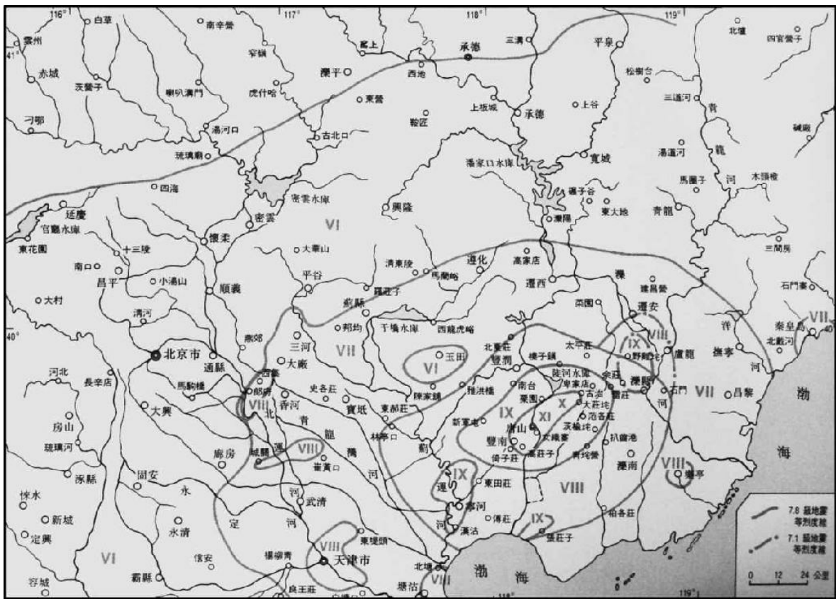
唐山地震等烈度线图
